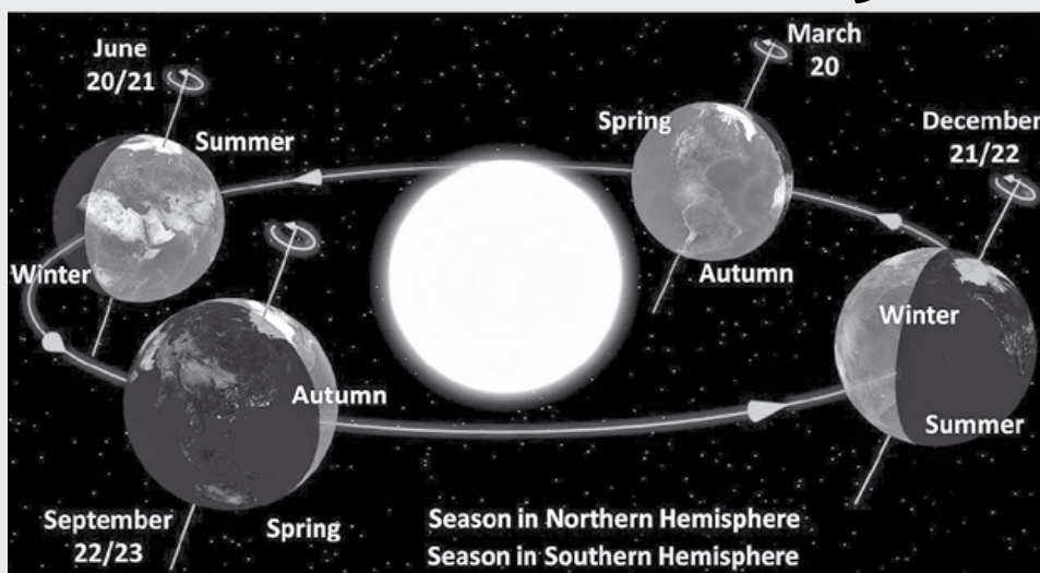
Διάγραμμα των γήινων εποχών του έτους όπως φαίνονται από τον Βορρά
